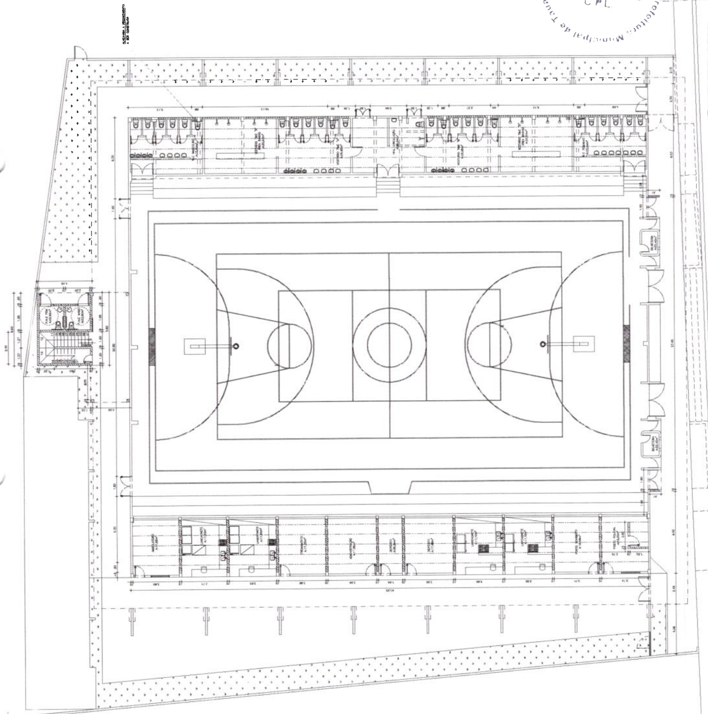
01) PLANTA REFORMA SUBSÓLO
