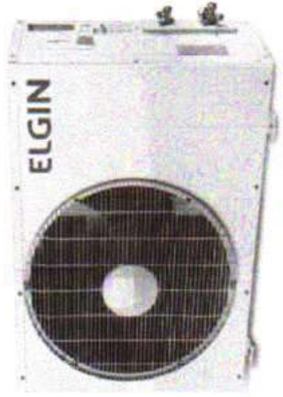
Proteção anticorrosão placa eletrônica com pintura de proteção contra umidade, corrosão e pó. Amarelamento e dureza da placa do ARO produto.
